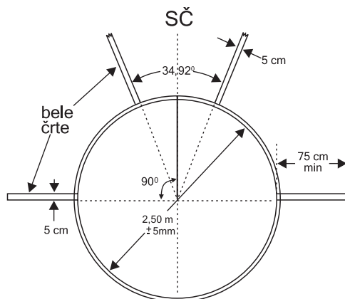
Tloris kroga za met diska
