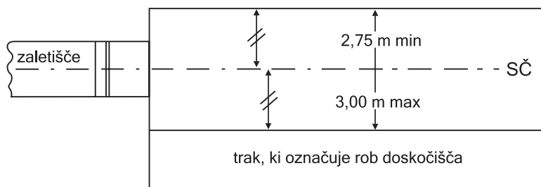
Središčnica doskočišča daljine/troskoka
