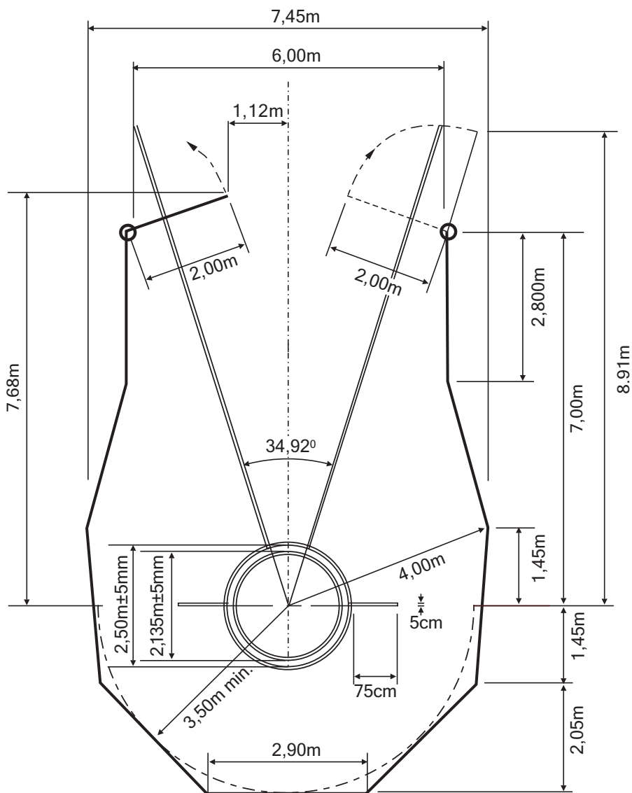
Zaščitna mreža za met kladiva in diska z vložkom Slika prikazuje položaj vrat za met kladiva pri metalcih desničarjih, črtkana vrata pa položaj pri levičarjih (dimenzije v metrih).
