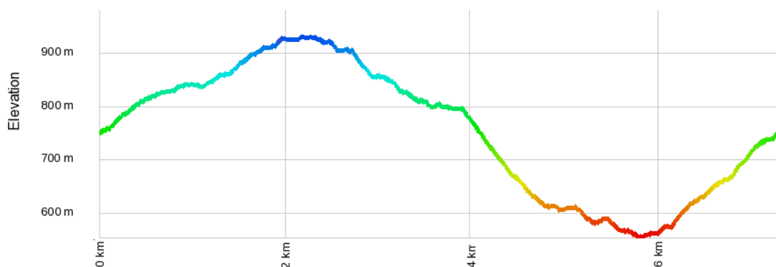
PROFIL TRASE
